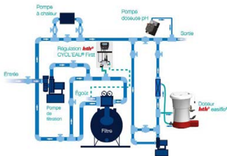
Schéma d'installation régulation ampérométrique hth® CYCL'EAU® FIRST avec un doseur hth® easiflo® SYSTEM
